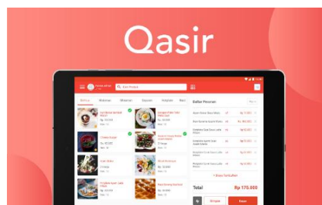
Gambar 5. Aplikasi Qasir
