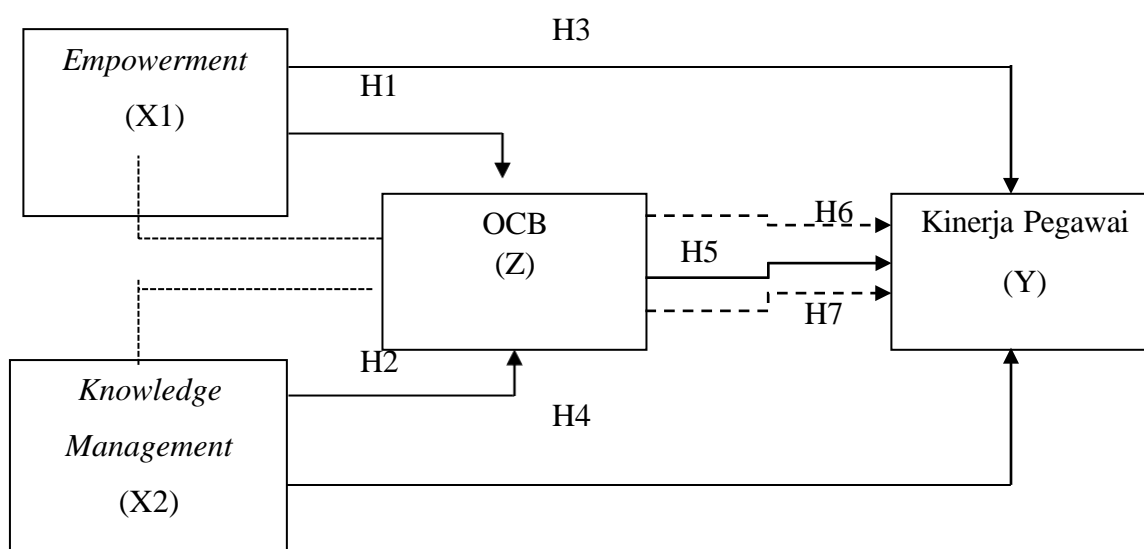
Gambar 1 Kerangka Pikir
